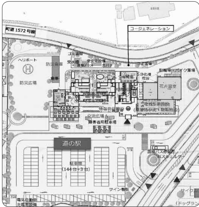
道の駅計画図
